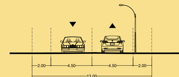
PROFIL EXISTENT A - A STR. PIATA VICTORIEI
