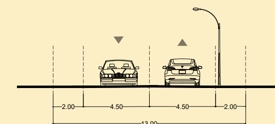
PROFIL EXISTENT A - A STR. PIATA VICTORIEI
