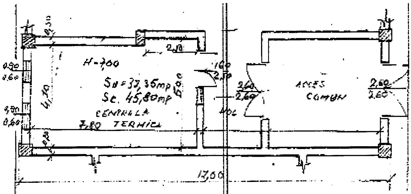
PLAN CENTRALĂ TERMICĂ
