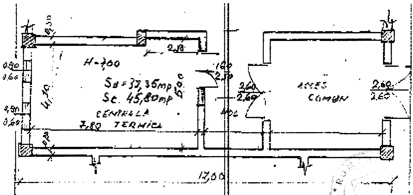
PLAN (PARȚIAL) AL FOSTULUI PUNCT TERMIC 2
